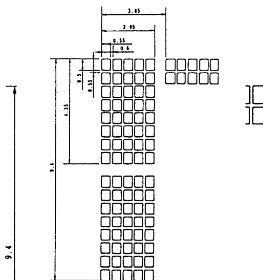
Fig. 2 Display pattern
